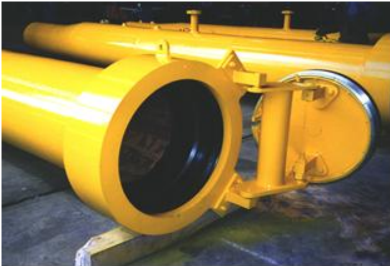
GASODUCTO GAS ANDES ARGENTINA – CHILE 9 TRAMPAS 24" x 20" #900
